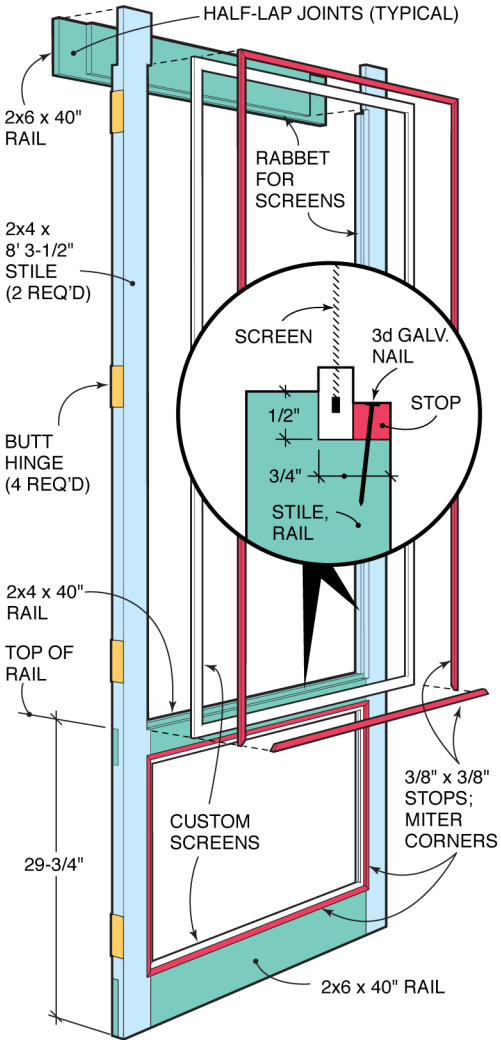
Fig. F Door Detail
