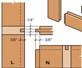
DOOR FRAME
