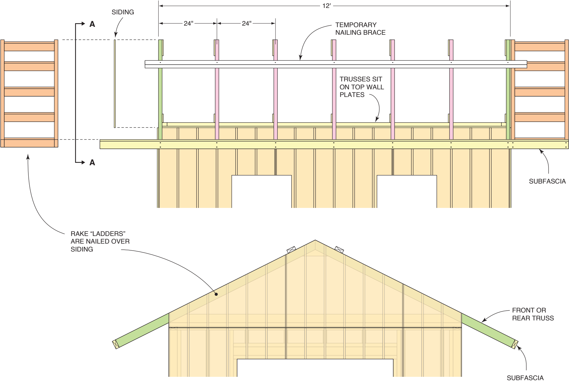
VIEW A-A
